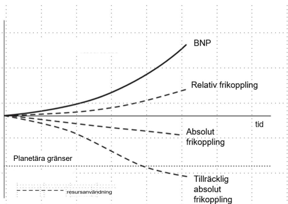
Figur 4 Illustration av relativ, absolut och tillräcklig absolut frikoppling. Från Raworth (2018).
